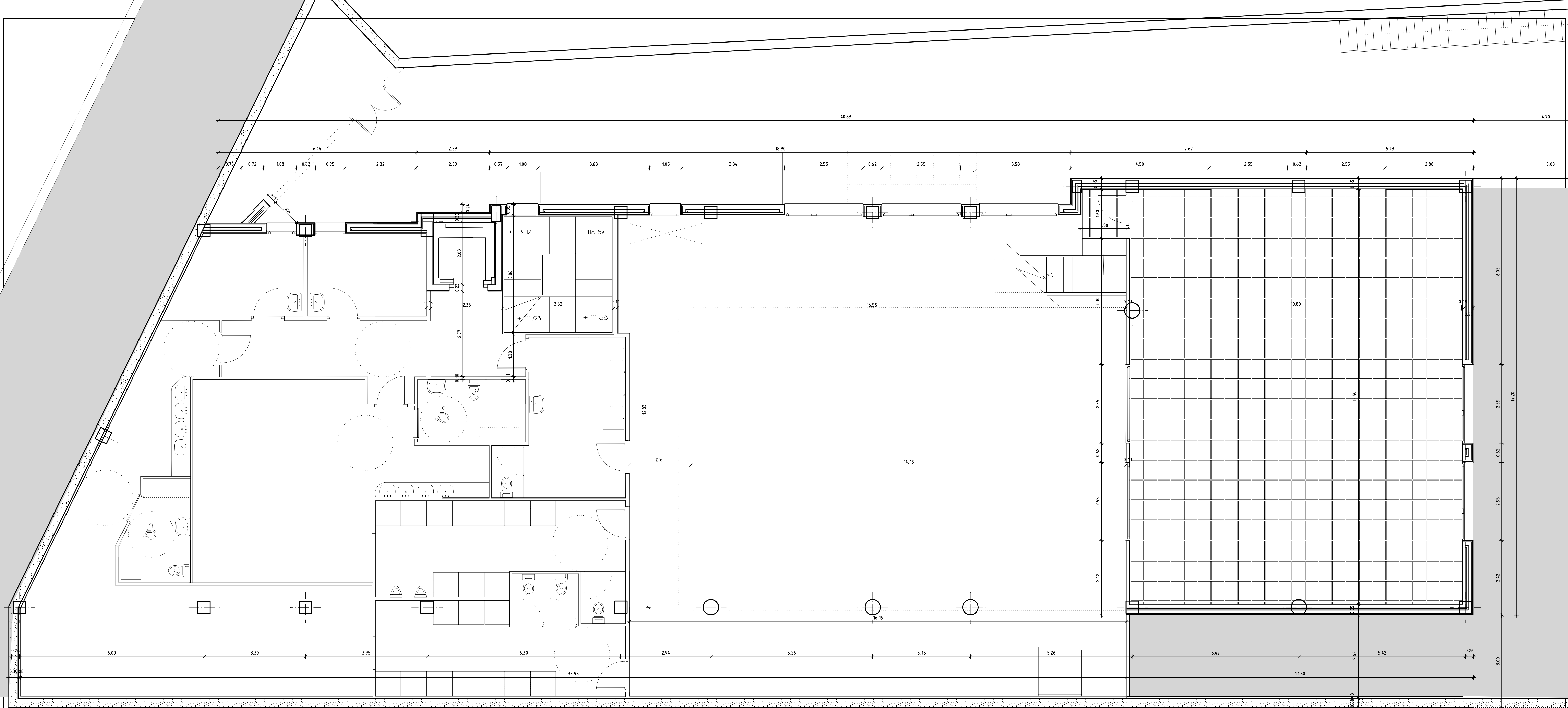
PLANTA SEMISOTANO
