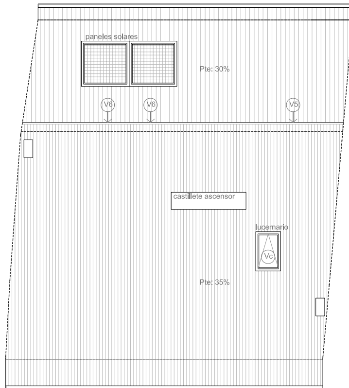
PLANTA CUBIERTA
