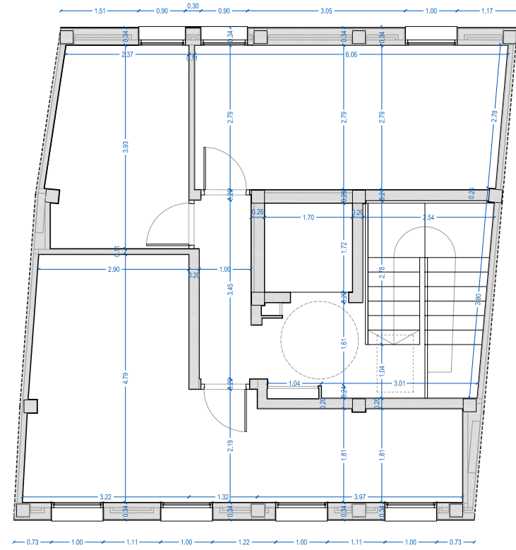
PLANTA BAJOCUBIERTA ACOTADA
