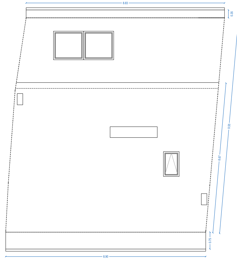
PLANTA CUBIERTA ACOTADA
