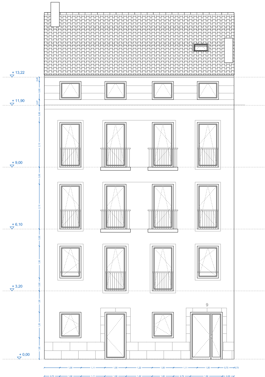
ALZADO PRINCIPAL. C/ RABAL 9.
